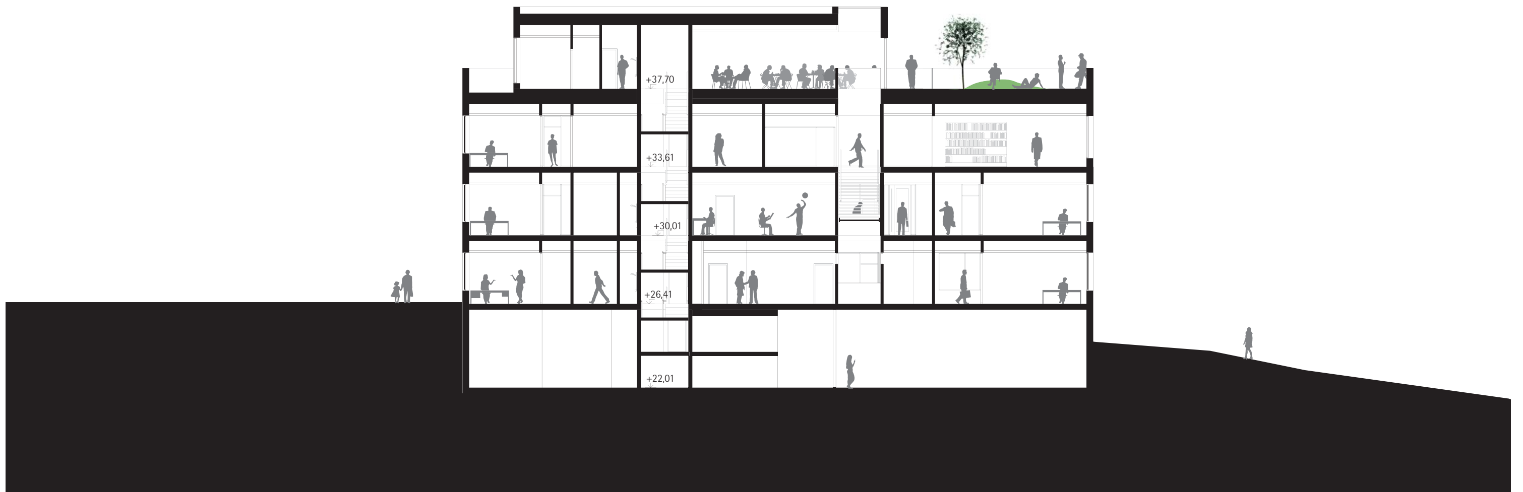
TVÄRSEKTION GENOM TILLBYGGNAD
